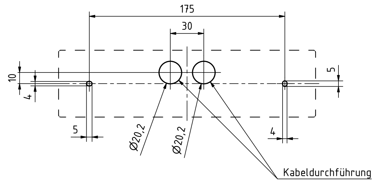
ALGOL 20 DA ( 1 : 2 )
