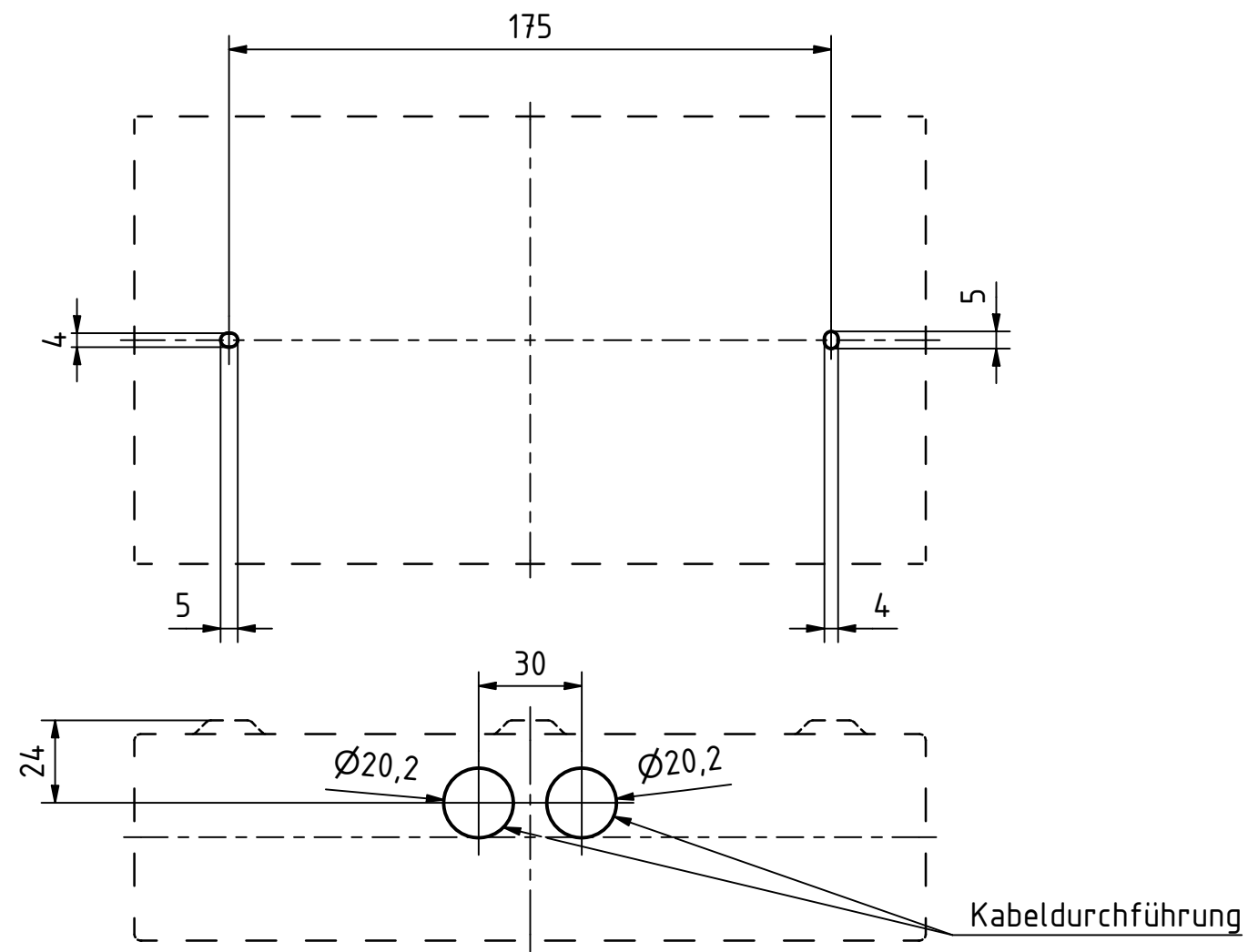
ALGOL 20 WA ( 1 : 2 )
