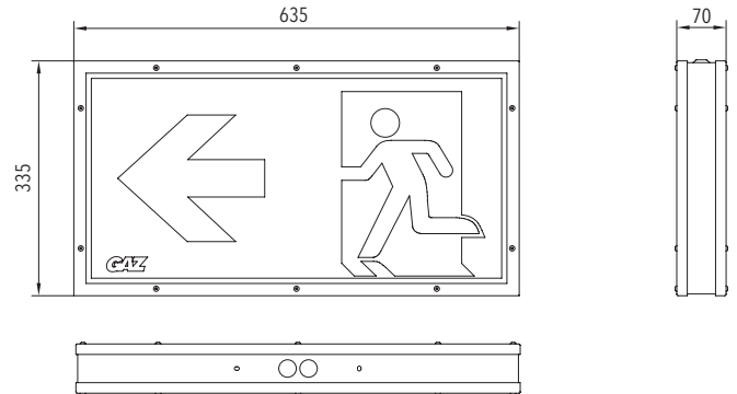
Deckenaufbau (DA) ceiling mounting (DA)
